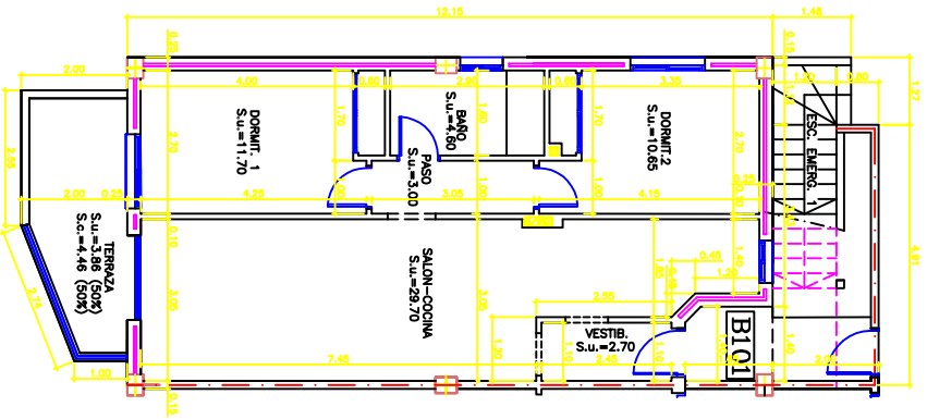
B-101. Planta cotas
