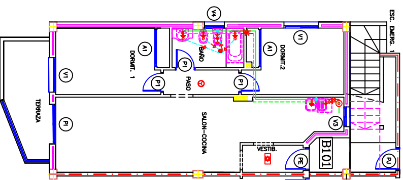
B-101. Planta inst fontanería
