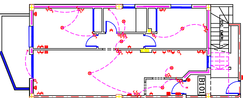
B-101. Planta inst eléctrica
