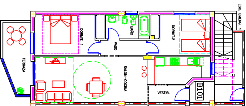
B-101. Planta mobiliario
