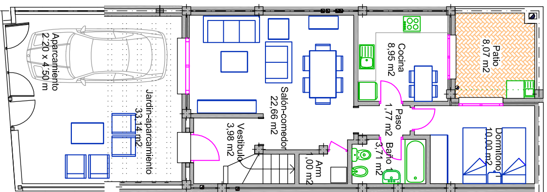
PRIMERA PLANTA
