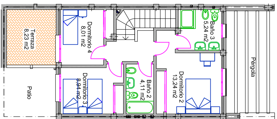
SEGUNDA PLANTA
