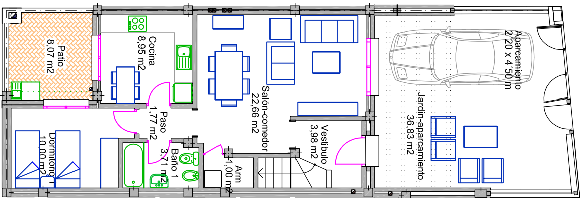
PRIMERA PLANTA
