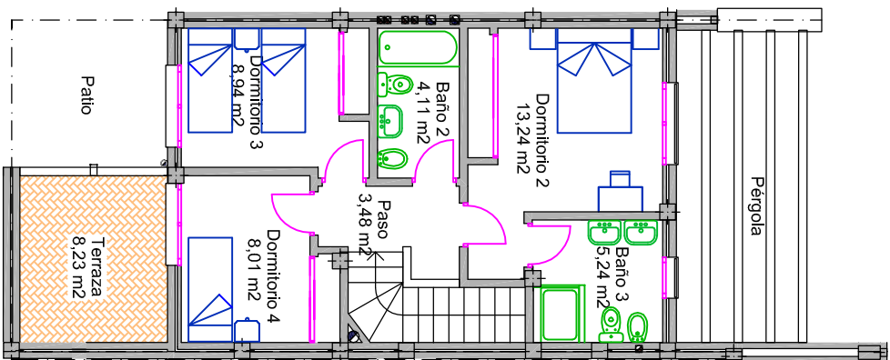
SEGUNDA PLANTA
